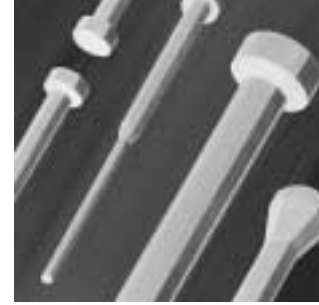
Schneidstempel HSS Form D, nach DIN 9861 Schaft und Kopf feinstgeschliffen
